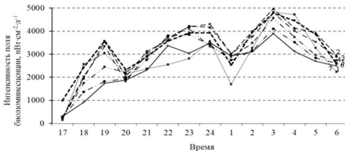
Рис. 1. Изменения интенсивности поля биолюминесценции в верхнем слое: 1 – 0-5 м; 2 – 5-10 м; 3 – 10-15 м; 4 – 15-20 м; 5 – 20-25 м; 6 – 25-30 м; 7 – 30-35 м.
